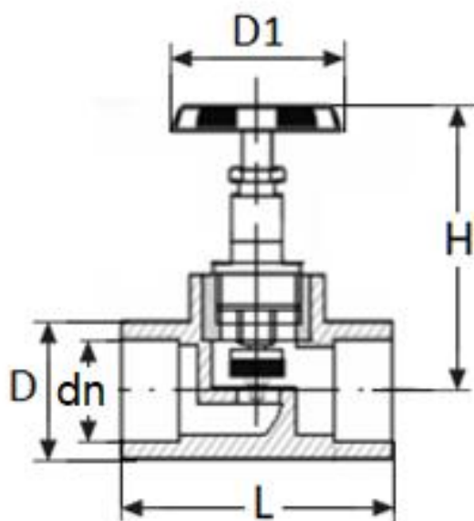
Рисунок 1- Вентиль прямой
