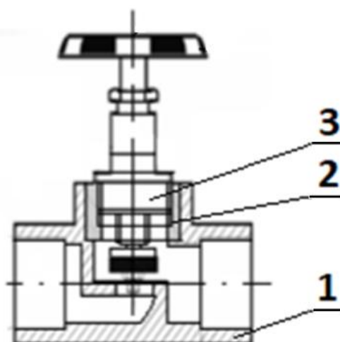
Рис.3 -Конструкция вентиля
