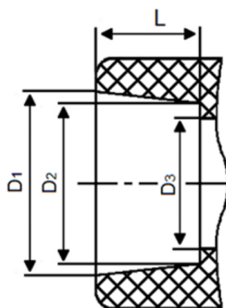
Рисунок 2- Раструбная часть фитингов
